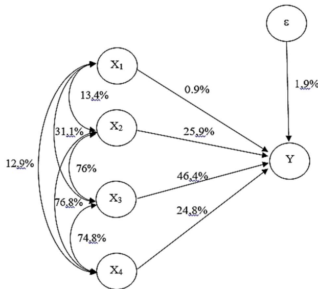
Gambar 1. Struktur Jalur Penelitian ( Path Analisis )
